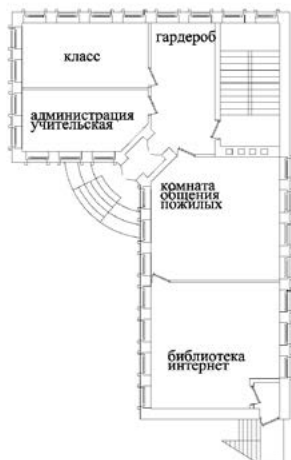
ПЛАН НА ОТМ. 0.00
