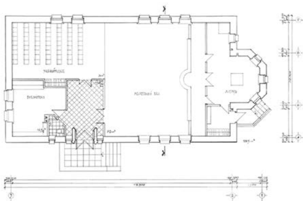
Проект воскресной школы в г. Всеволожске
