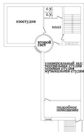
ПЛАН НА ОТМ. 6.0
