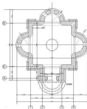
Рис. 3. Храм-часовня. Планы, разрез, восточный фасад. Вариант с подвалом.
