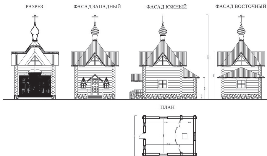
Рис. 1. Храм-часовня из цилиндрованного бревна. План, разрез, фасады.
