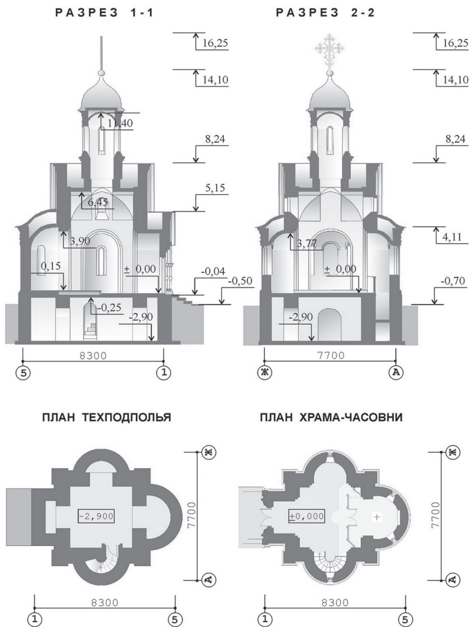
Рис. 6. Храм-часовня. Фасады, разрезы, планы. Вариант с трехлопастным восьмискатным покрытием.
