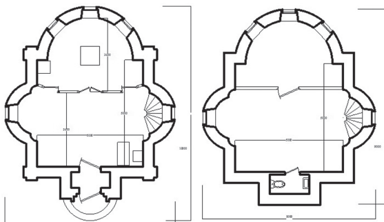
Рис. 5. Храм-часовня. Планы. Вариант с алтарной апсидой и винтовой лестницей в под- вал, расположенной в боковой экседре.
