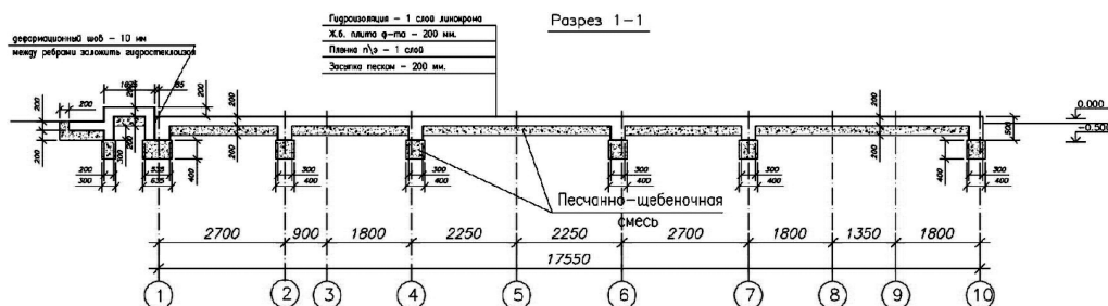
Разрез фундаментной плиты
