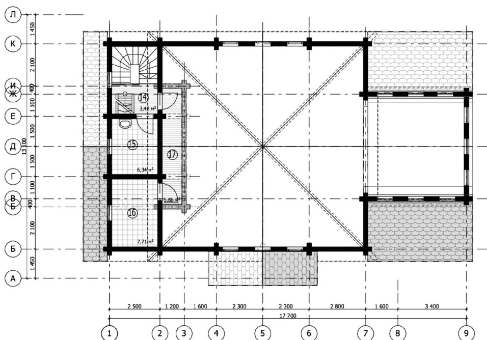
План второго яруса
