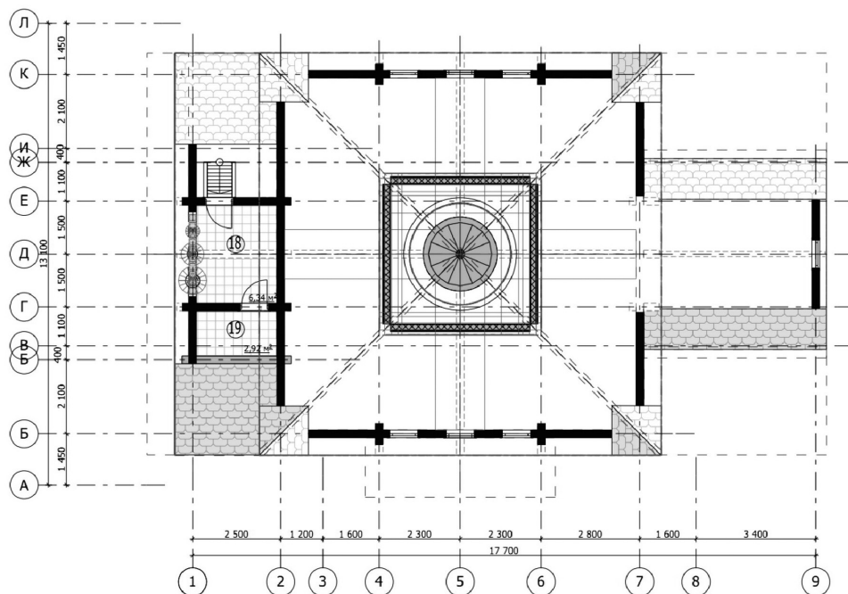
План третьего яруса
