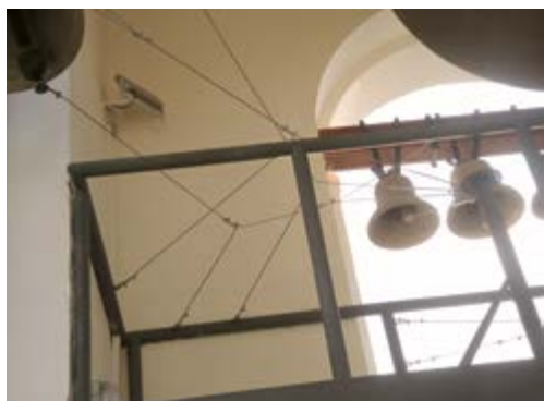
Система настроенных тяг и оттяжек для управления колоколами: тяги идут под выверенными углами
